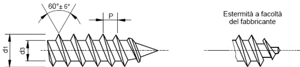
Dimensioni delle filettature dimensioni in mm
