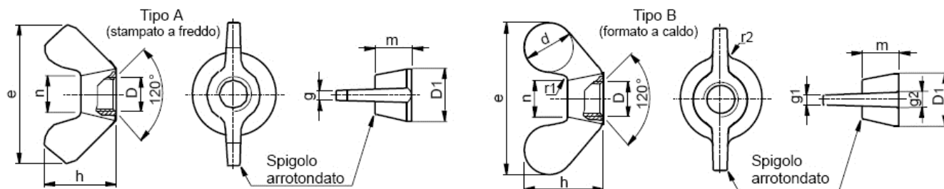
Tipo A stampati a freddo
